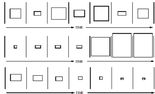
Abb. 3.6: Entwicklungstypen: (von oben) Pulsar, Supernova, Weißer Zwerg
