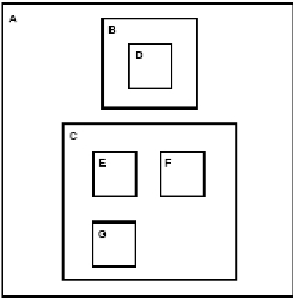
Abbildung 2 Verschachtelter Graph [97]
