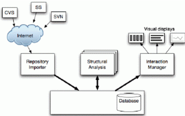
Abb. 4.1: Augur-Architektur
