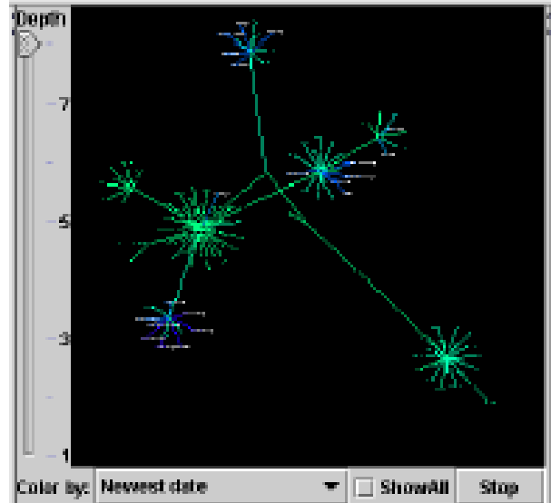
Abb. 4.3: Sekundärsicht: Graphendarstellung
